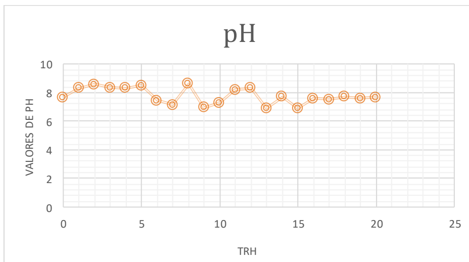
Gráfica 1. Variación de pH en el reactor de biodiscos
