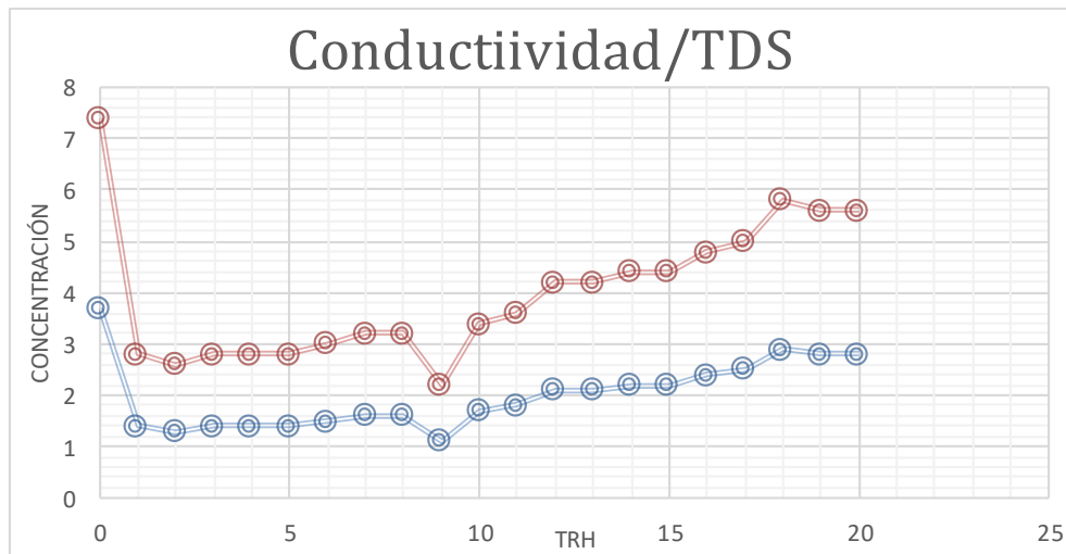
Gráfica 3. Variación de Conductividad/TDS en el reactor de biodiscos.
