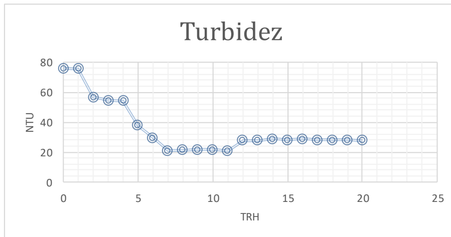
Gráfica 2. Variación de la turbiedad en el reactor de biodiscos
