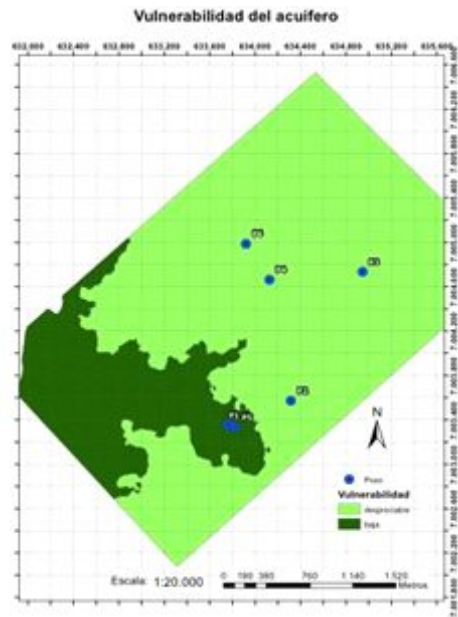
Figura 4. Vulnerabilidad a contaminación al acuífero según el modelo GOD (Foster et al. 2002), Los pozos 1 y 5 se encuentran en la categoría "baja", mientras que los pozos 2, 3, 4 y 6 se encuentran en la categoría "despreciable".
